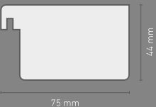
Aufbau Blendrahmen Blind frame construction
