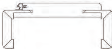
Furnierte Softzarge FS 60 mm Bekleidung abgerundet R5, ohne Profil Bekleidungen auf Gehrung
