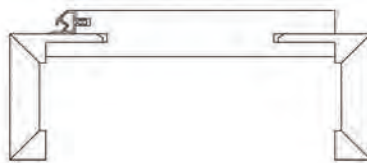
Furnierte Softzarge FE 60 mm Bekleidung eckig, ohne Profil Bekleidungen auf Gehrung
